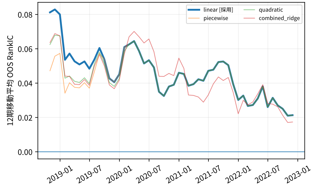
FA3002 売上成長率 | 採用=linear
