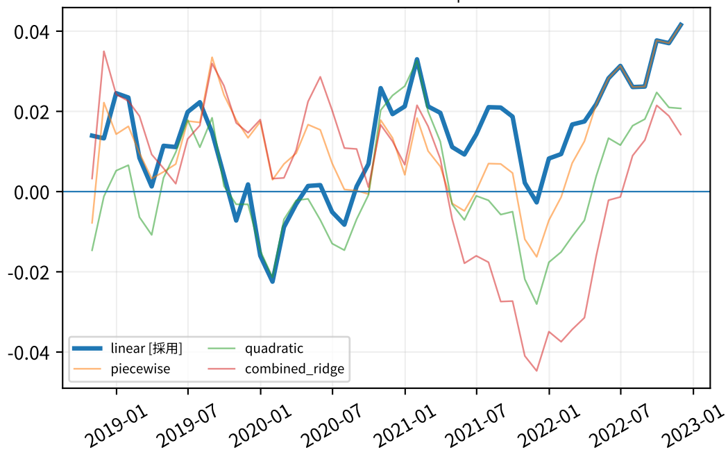
FA1001 12か月モメンタム | 採用=linear
